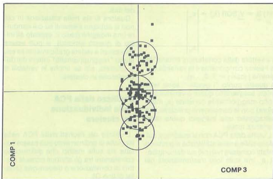
Figura 8 - Esempio di output grafico di un caso reale, dove il modello comprendeva 22 variabili e 172 campioni. Si aveva modo di presumere l'esistenza di quattro raggruppamenti interni, clusters, che sono quelli individuati dai cerchi. La rappresentazione è stata fatta nello spazio della 1' e 3' c.p. . Come si vede nella realtà le situazioni non sono mai chiarissime. I dati sono gli stessi della figura 7.
